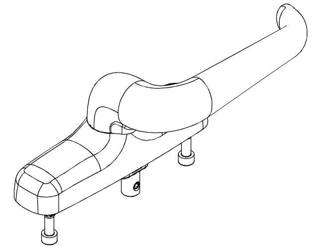
Vista isometrica Scala: 1:2
